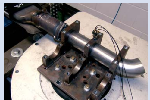
Prüfung von Abgasanlagen bei ArvinMeritor Emissions Technologies GmbH in Augsburg
