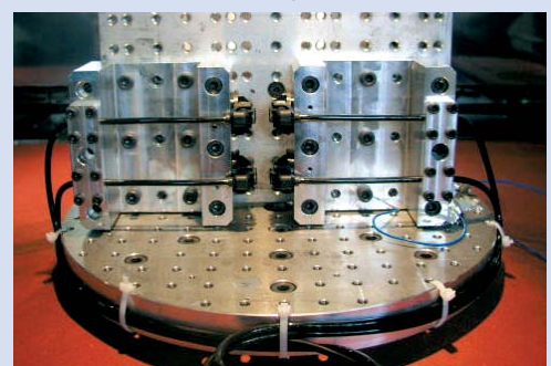
Schwingprüfung von Kfz-Steckverbindern, Hirschmann Automotive GmbH, Rankweil/Österreich
