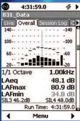
Fig. 12 1/1 Octave Display
