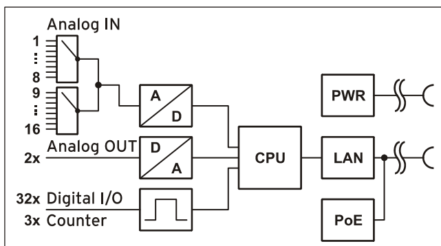
Funktionsschaltbild
